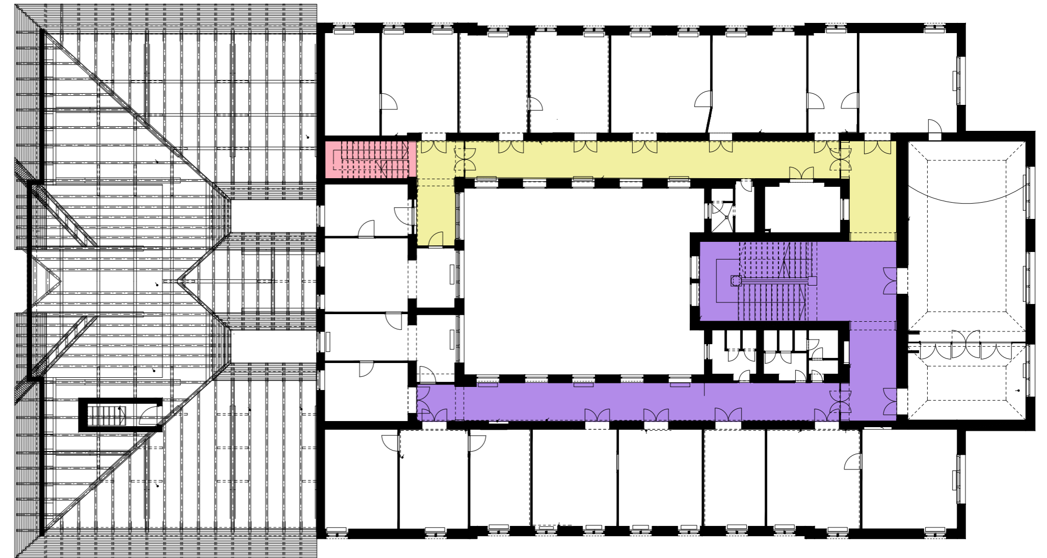
ÁTTEKINTŐ 2. EMELETI ALAPRAJZ
