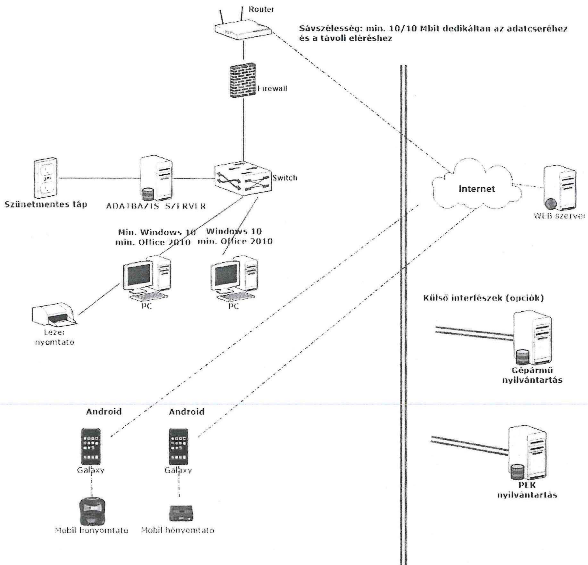
Közrend IT rendszer topológiája
